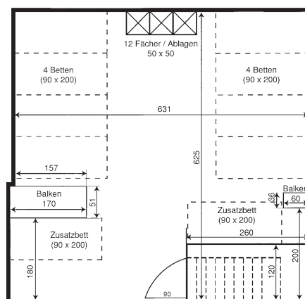
Grundriss Dachgeschoss
